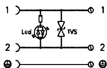
bipolare LED und Schutzbeschaltung Transil-Diode
