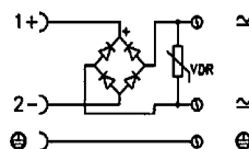
Brückengleichrichter, und Varistor
