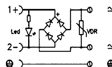
Brückengleichrichter, LED Anzeige und Varistor
