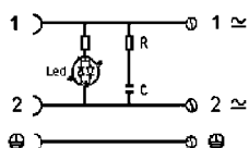
bipolare LED und RC Schutzbeschaltung
