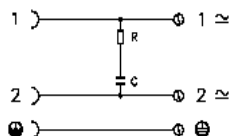
RC-Schutz- beschaltung
