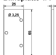
Blindplatte 1/4"
