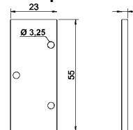
Blindplatte 1/8"
